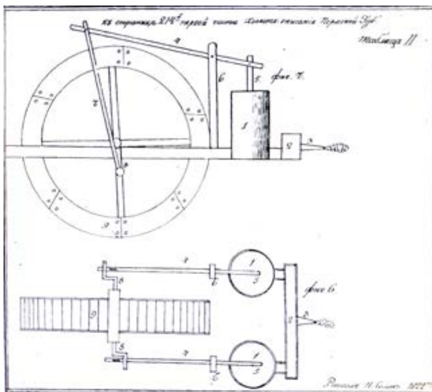
Рис. цилиндр мехов 1803 г.
